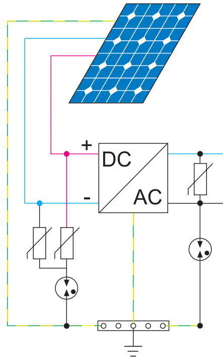
Рис 10: Пример фотогальванической системы для здания, не оборудованного системой защиты от молний; защита со стороны DC при помощи УЗИП с U_{ocstc} = 420 В, и защита со стороны AC устройством 7P22, характерным для систем TT.
